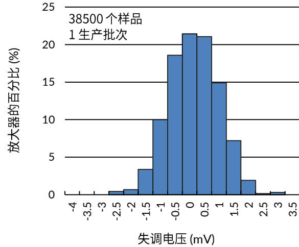
图 14. 失调电压分布, V_S = \pm 2.5\text{V}
