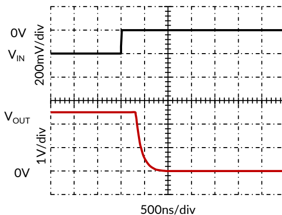
图 12. 正向过载恢复， V_S = \pm 2.5\text{V} ， G = -100
