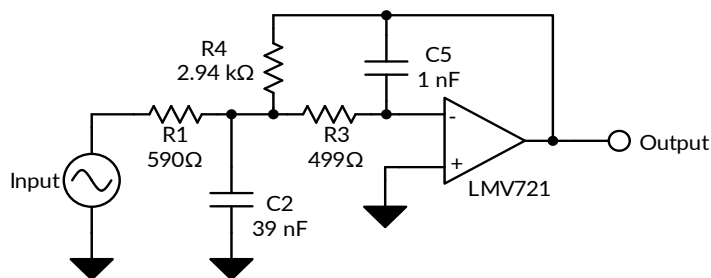
图 18. 25-kHz 低通滤波器
