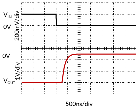
图 13. 反向过载恢复, V_S = \pm 2.5\text{V} , G = -100
