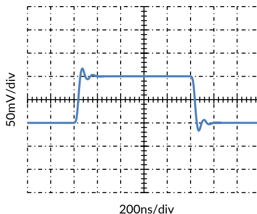
图 10. 小信号阶跃响应， C_L = 100\text{pF}
