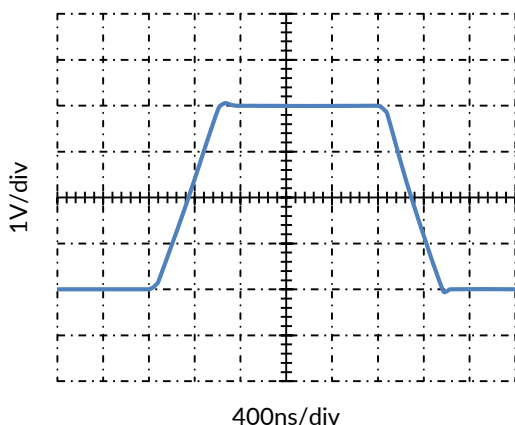
图 11. 大信号阶跃响应， C_L = 100\text{pF}
