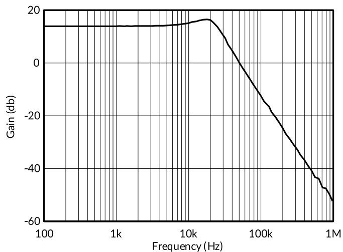
图 19. 低通滤波器
