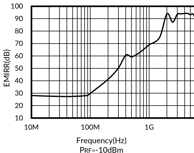
图 16. LMV721 EMIRR 和频率的关系
