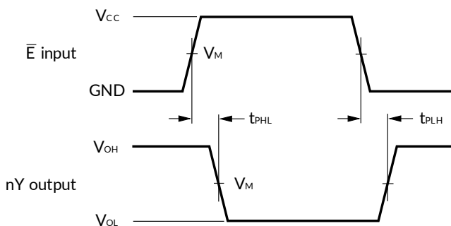
图 2. 输入 ( \bar{E} ) 到输出 (nY) 的传播延迟
