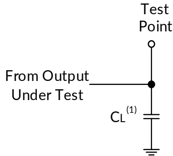
图 1. 用于推挽输出的负载电路
