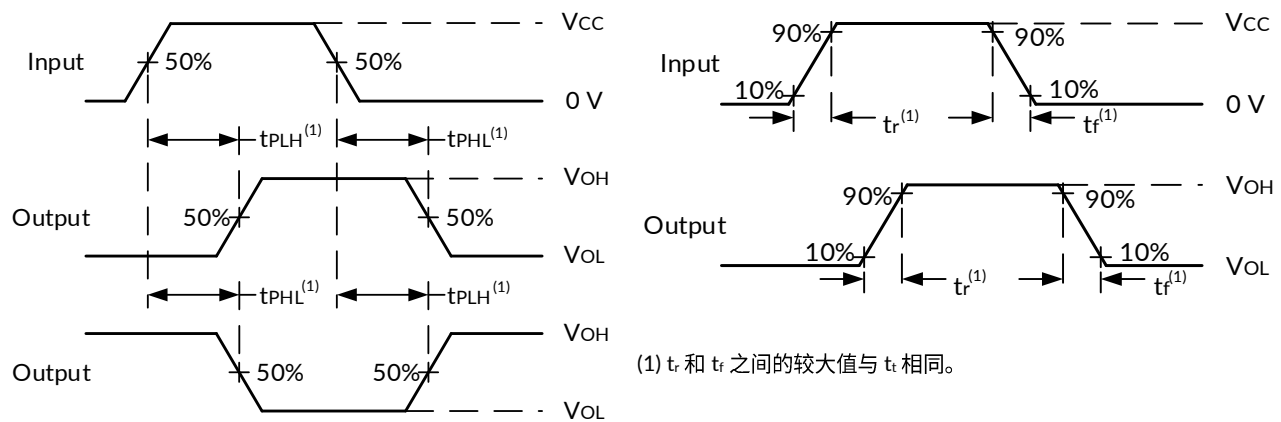
图 3. 标准 CMOS 输入的电压波形、输入和输出转换
