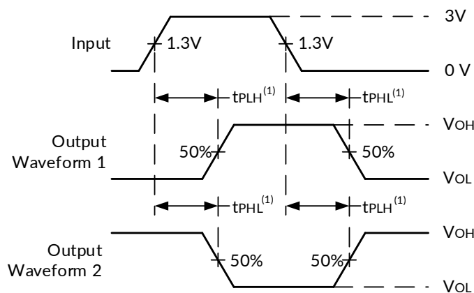
图 2. 标准 CMOS 输入的电压波形、传播延迟
